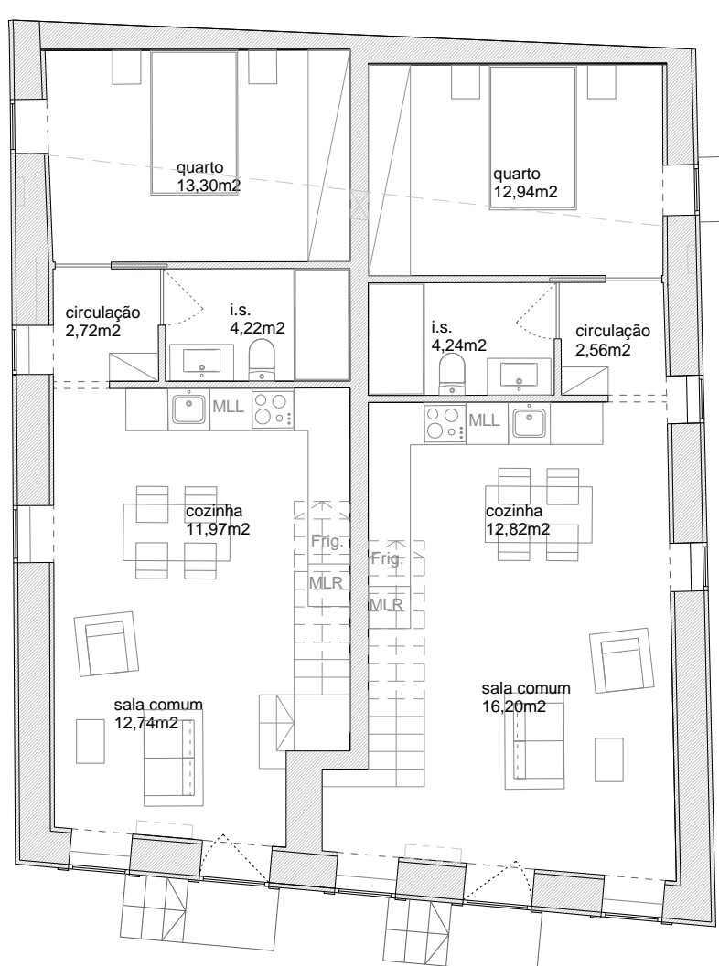
Planta rés-do-chão
