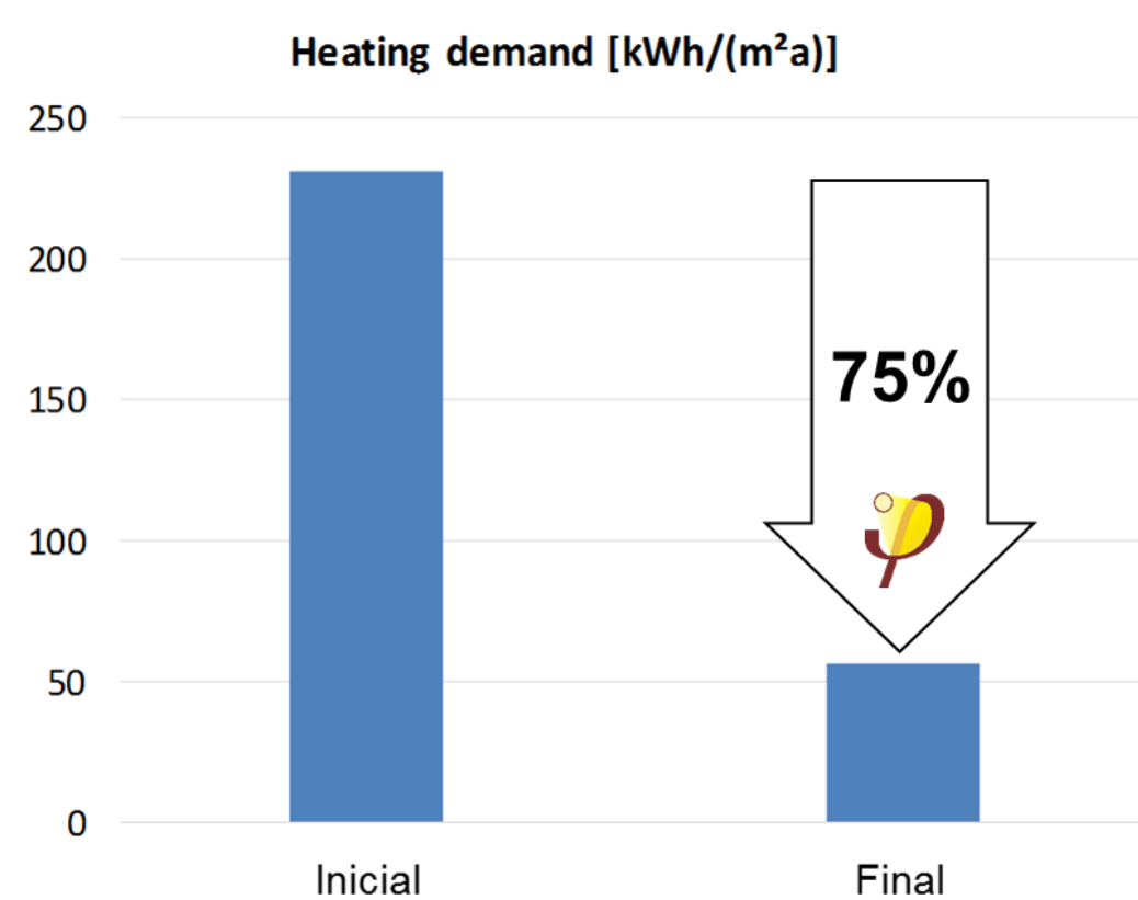
Comparação das necessidades de aquecimento © Homegrid
